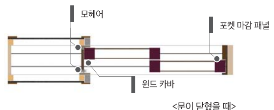
<문이 닫혔을 때>
