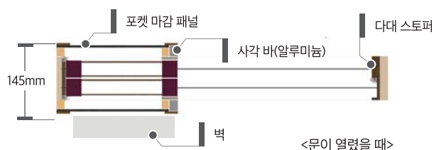
<문이 열렸을 때>
